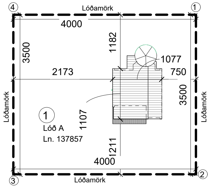
1 Afstöðumynd 1 : 500
