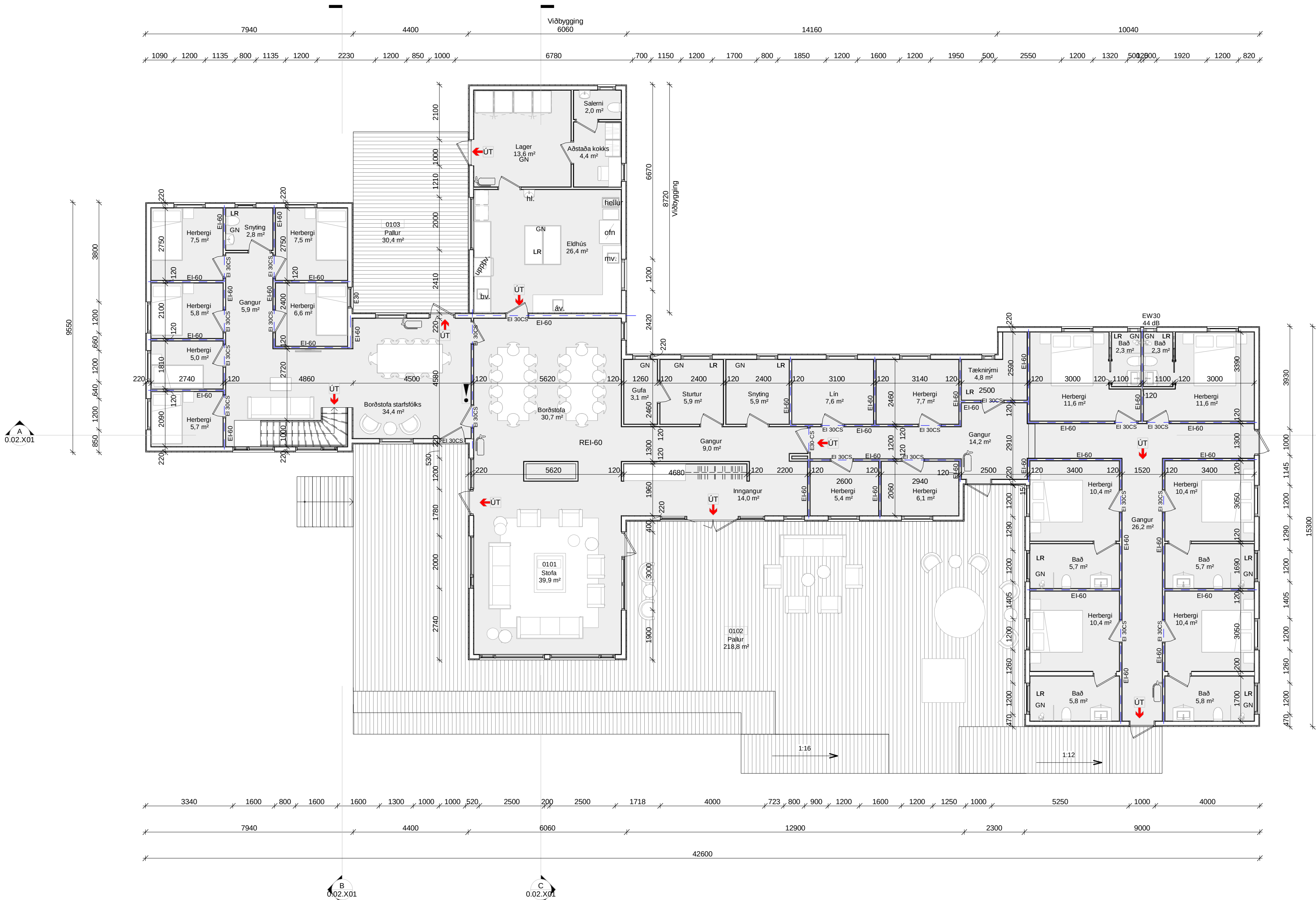
GRUNNMYND - 1. HÆÐ 1 : 100
