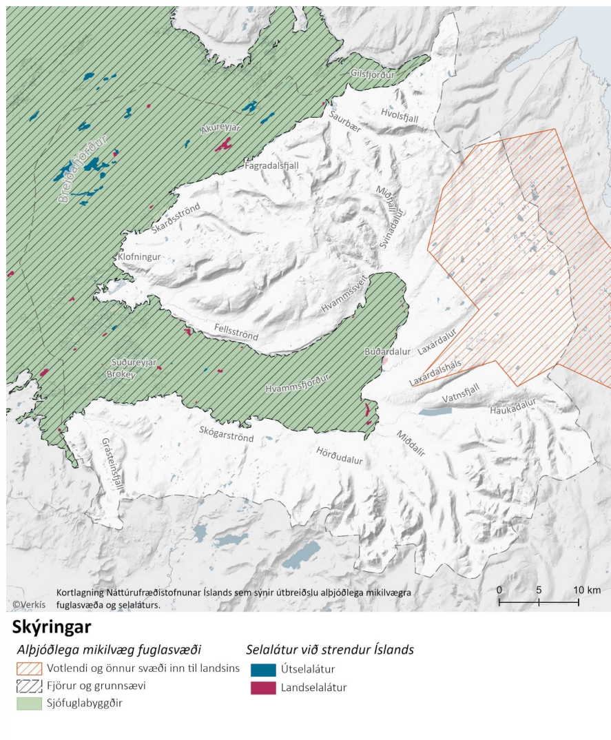
Mynd 3.9 Mikilvæg fuglasvæði og selalátur í Dalabyggð.
