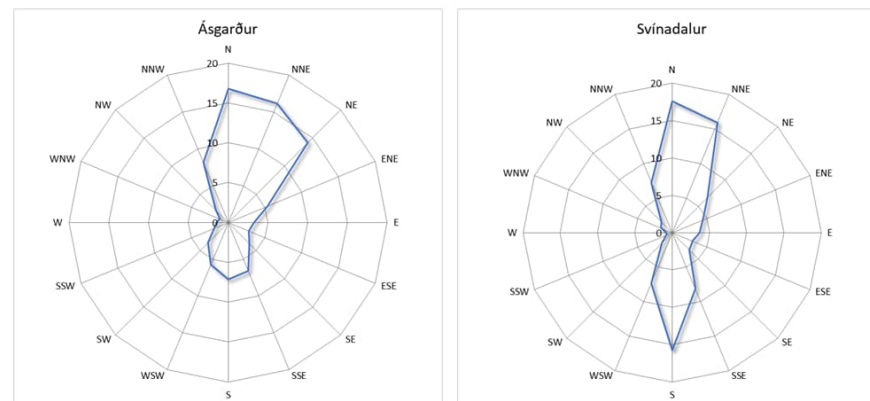
Mynd 3.5 Tíðni vindátta í Ásgarði og Svínadal, meðaltal árána 2010-2019. 6
