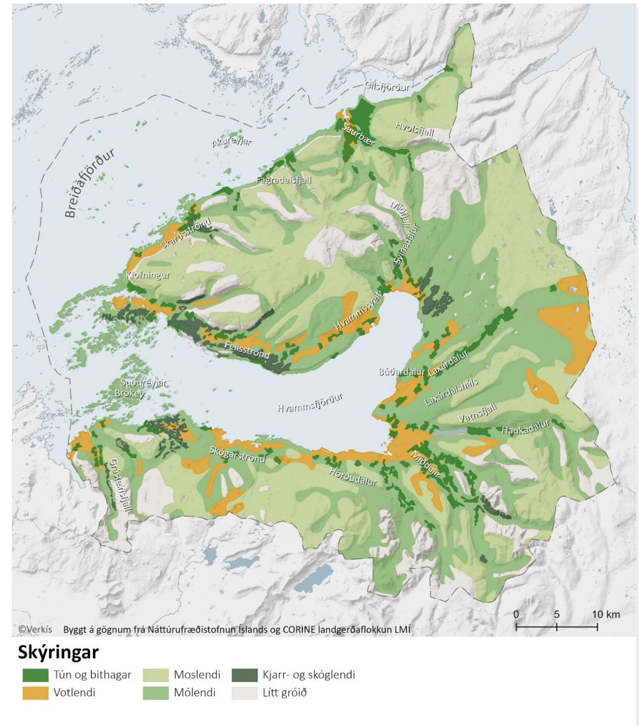
Mynd 3.8 Gróðurfar í Dalabyggð
