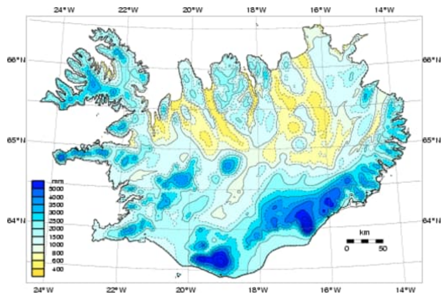
Mynd 3.6 Meðalúrkoma ársins 1971-2000.
