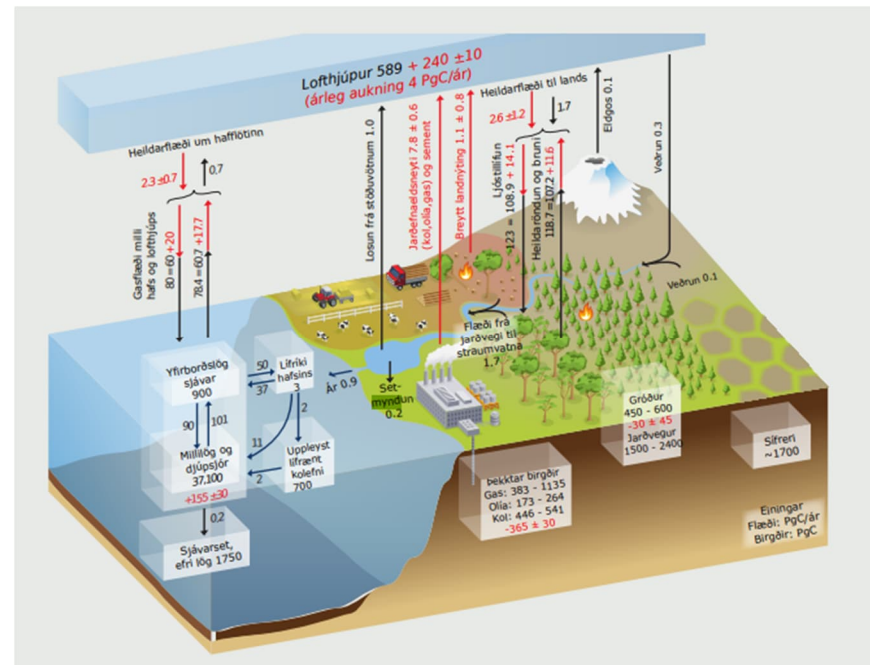
Mynd 4.1 Einfölduð mynd af kolefnishringrás jarðar 2000–2009. Úr skýrslu vísindanefndar um loftslagsbreytingar um áhrif loftslagsbreytinga á Íslandi.
