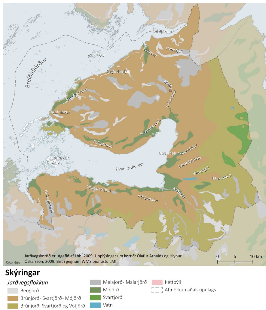
Mynd 3.7 Jarðvegskort af Dalabyggð.
