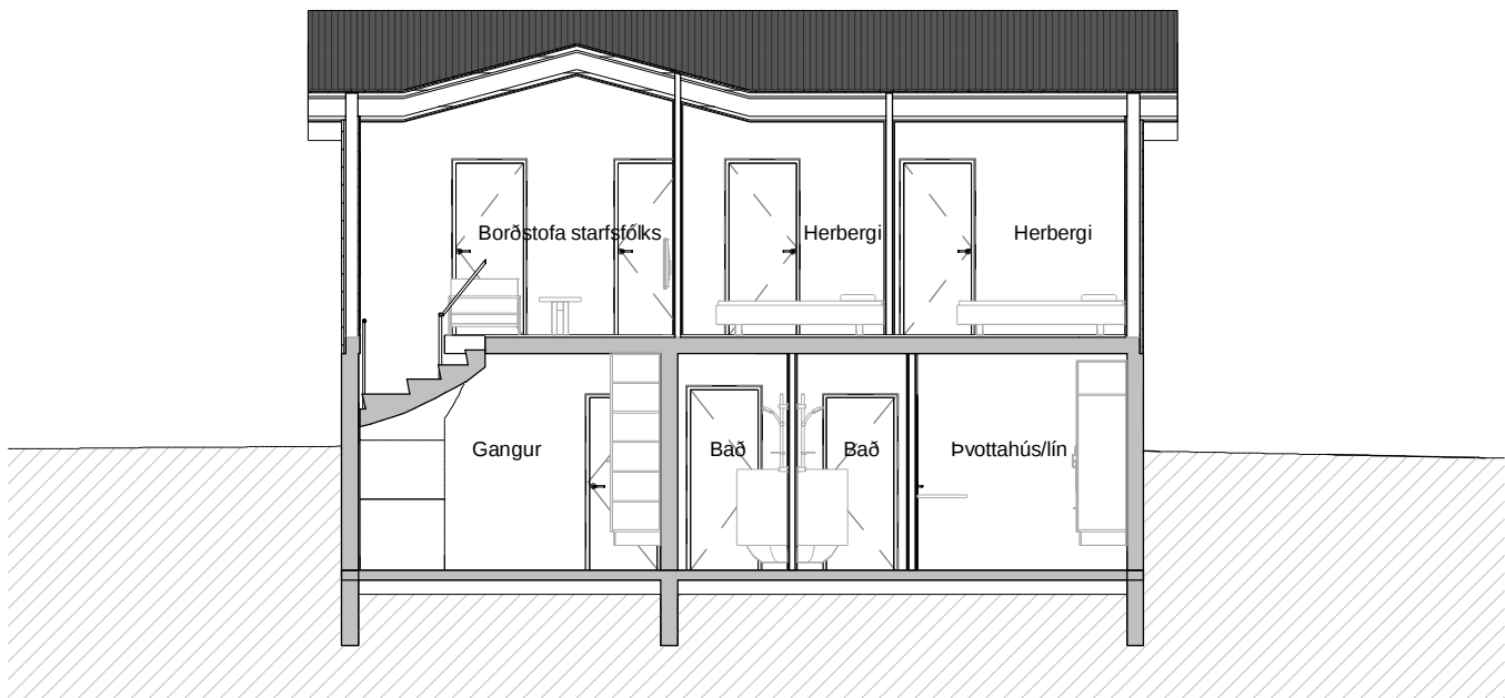
B Snið B-B 1 : 100
