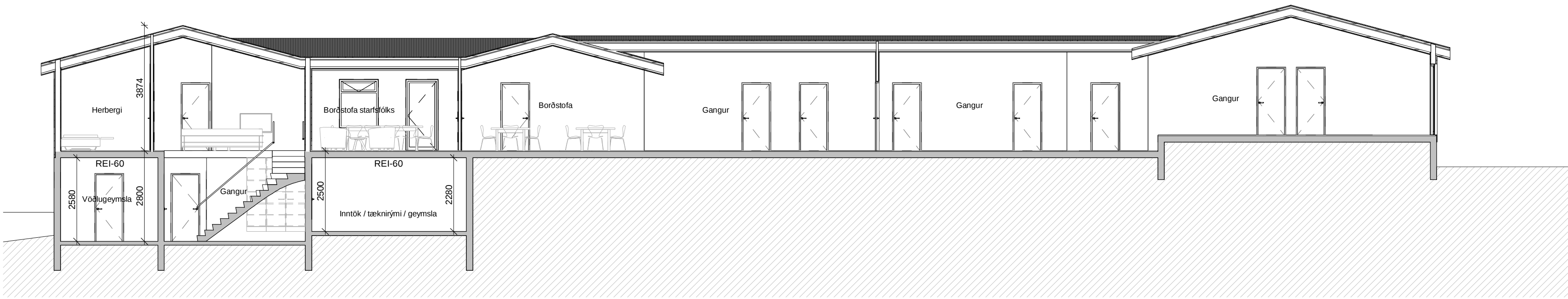
A Snið A-A 1 : 100
